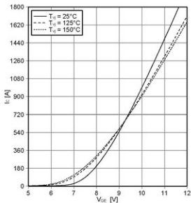
Übertragungscharakteristik IGBT-Chopper (typisch) transfer characteristic IGBT-Chopper (typical)
